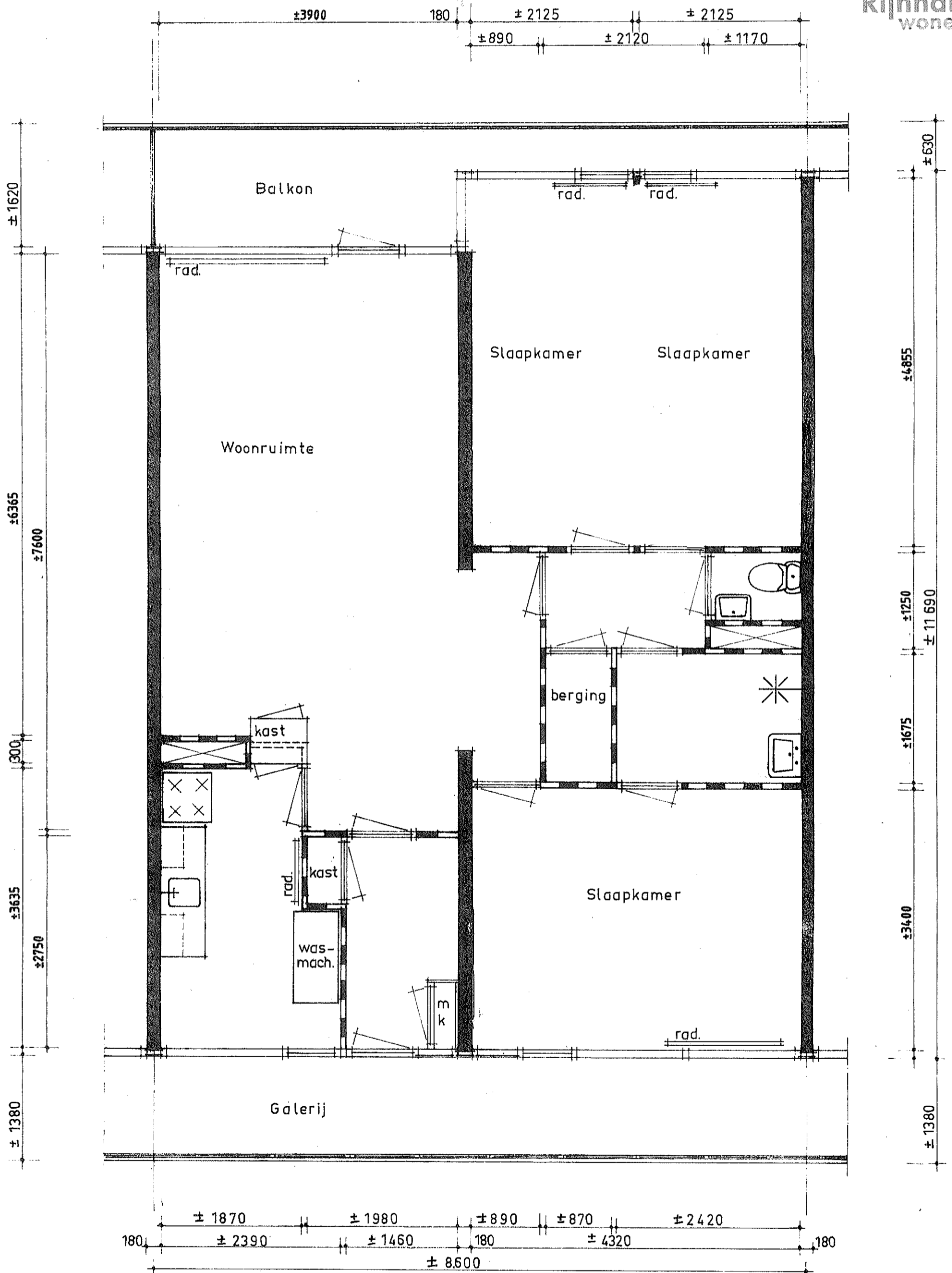
Plattegrond 1:50
