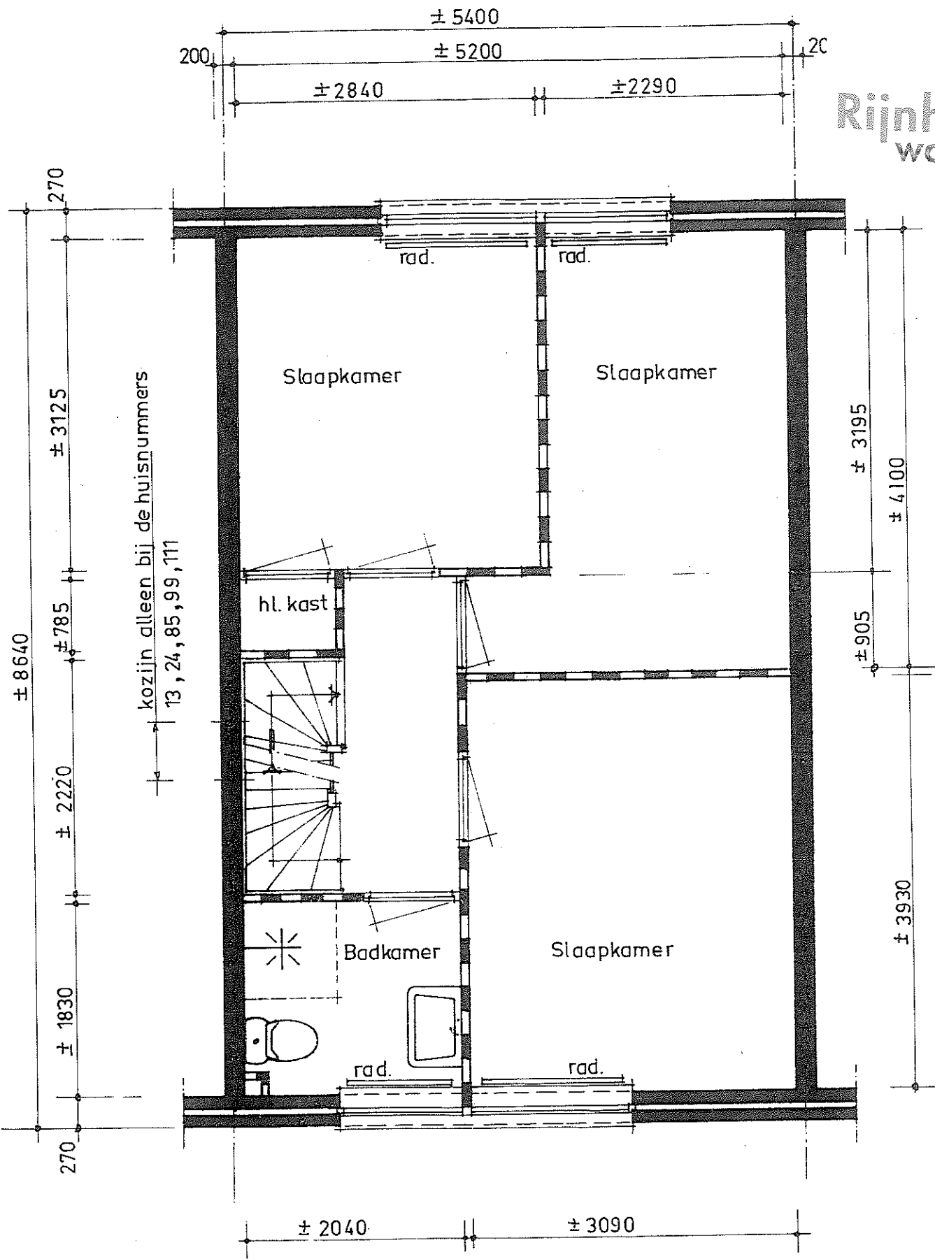
Slaapverdieping 1:50
